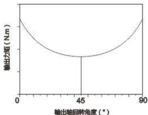
双作用输出力矩特性
