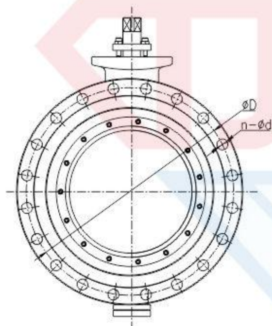
600LB阀体端面法兰连接尺寸
