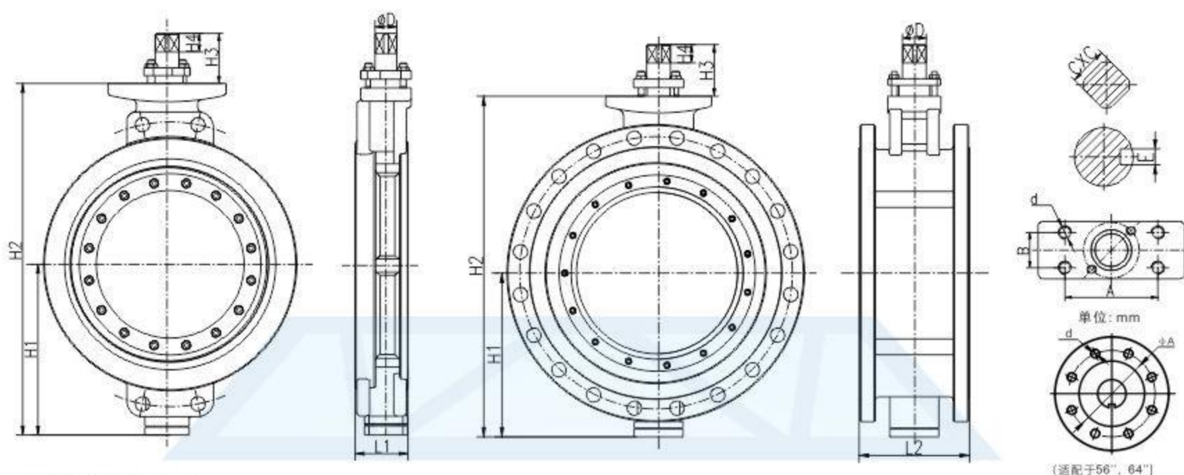
阀体结构尺寸
