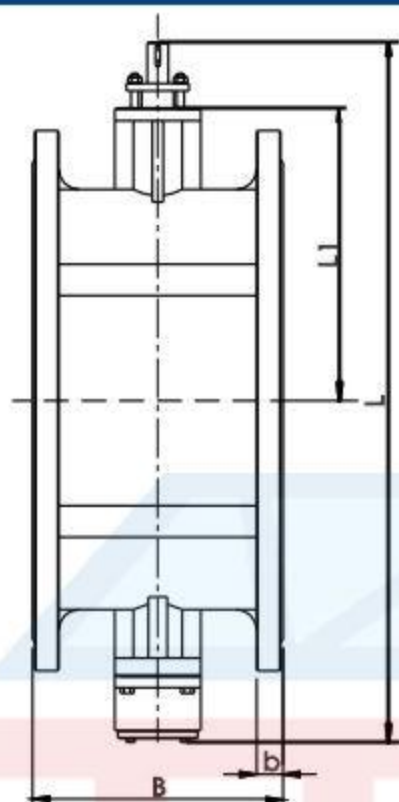
阀体结构尺寸(PN0.25/0.6)
