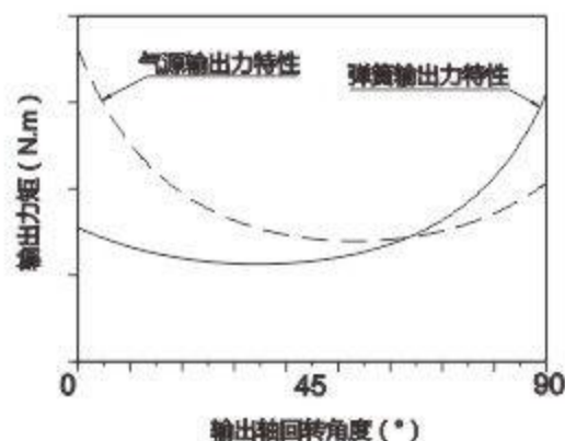
单作用气开输出力矩特性(气源0.5MPa)
