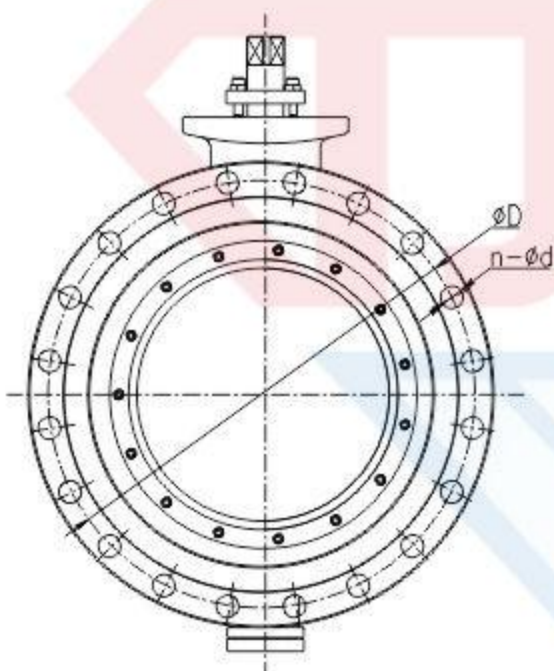
PN4.0阀体端面法兰连接尺寸
